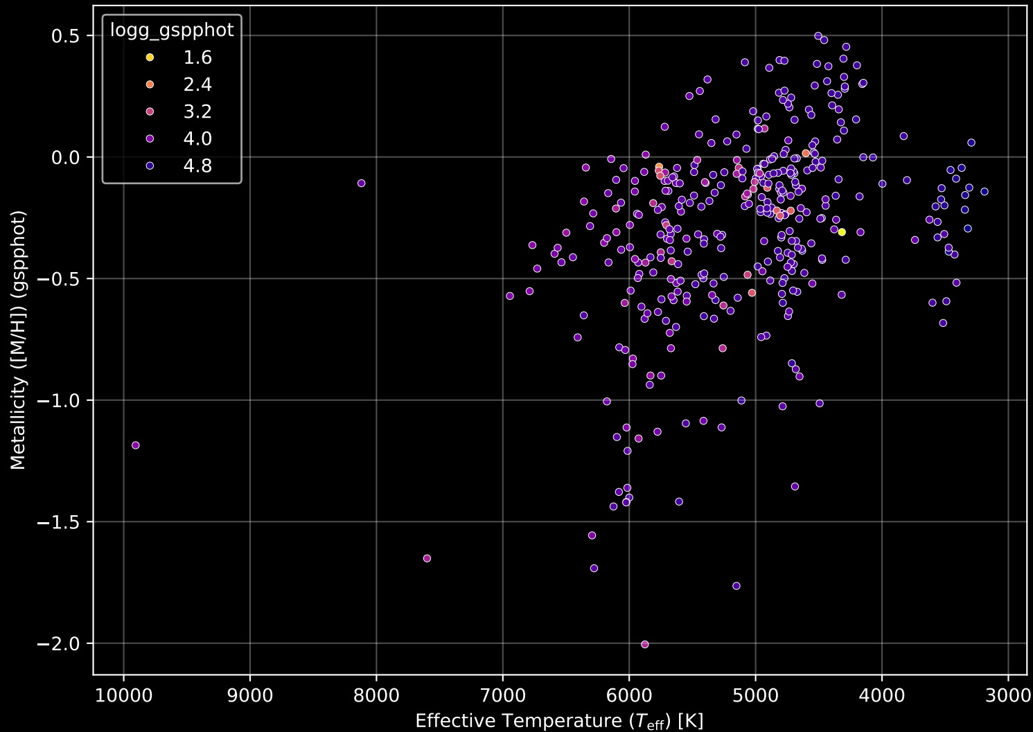
APOGEE DR17 Field: [GD1-5] Stellar Population Parameters (n= 376)
